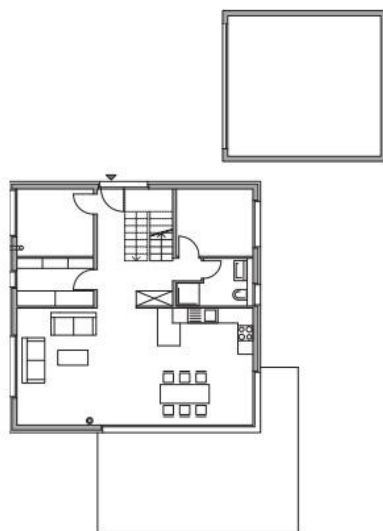
🕒 Niveau 0
