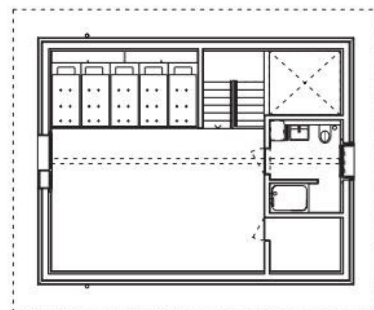
Niveau +2
