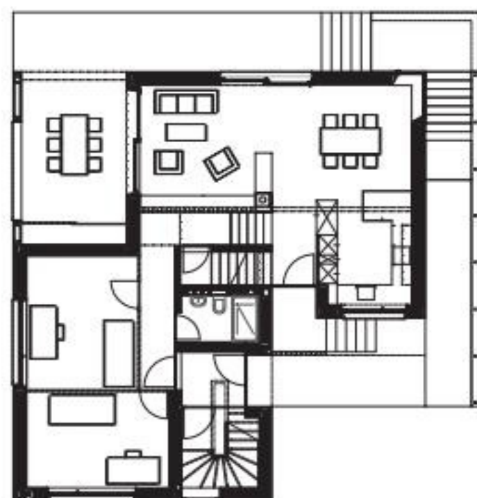
① Niveau 0
