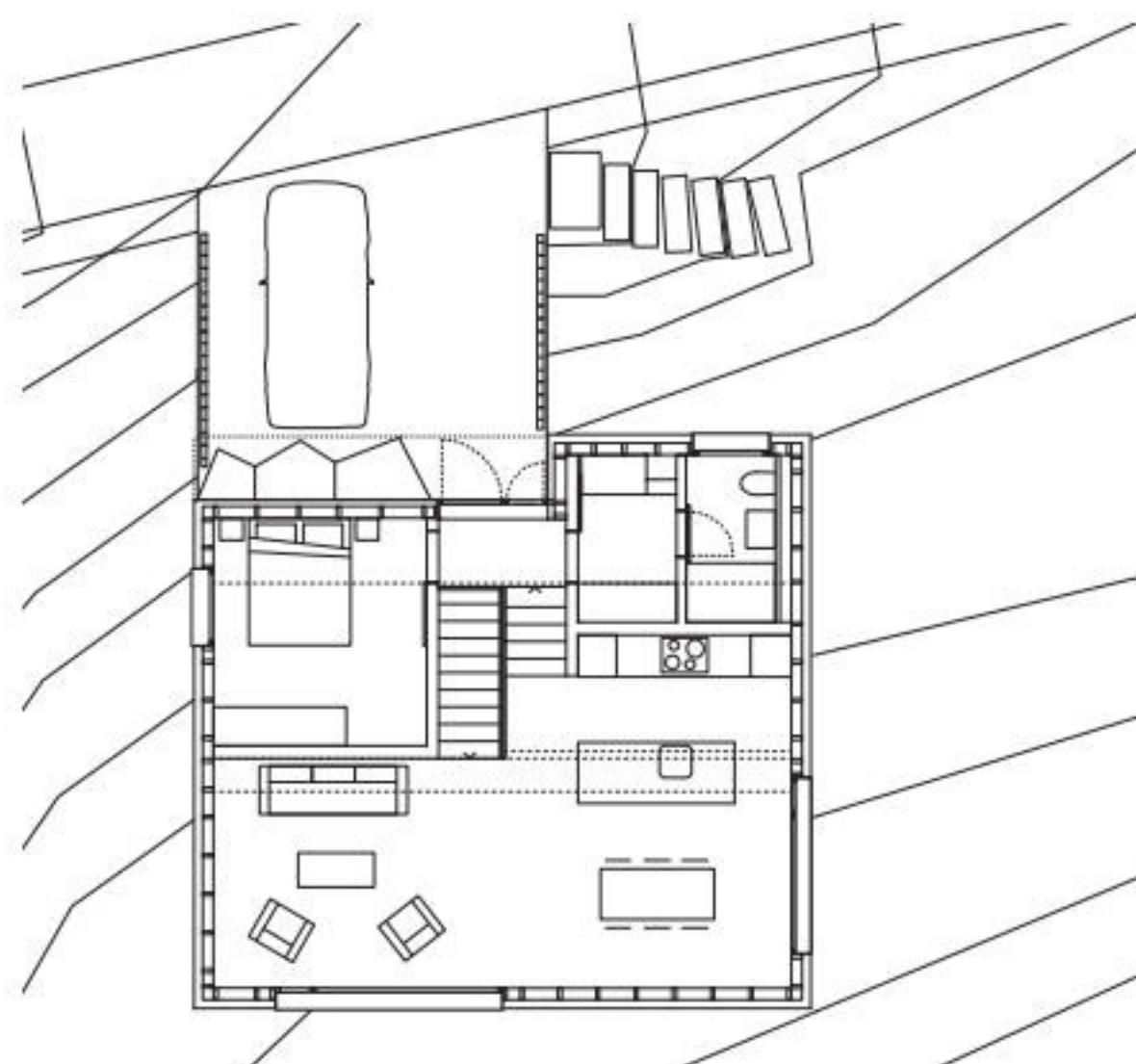
Niveau 0
