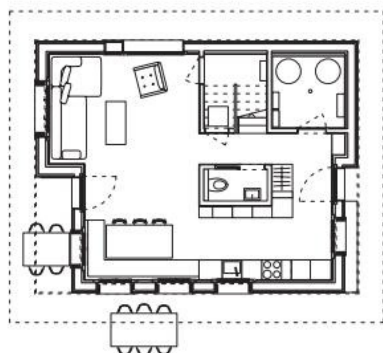
Niveau 0
