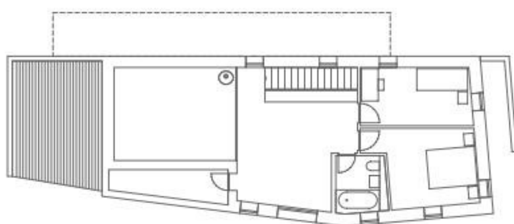
Niveau +1
