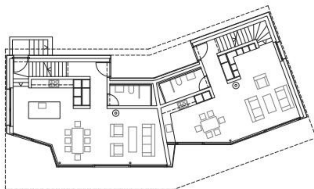
🕒 Niveau 0
