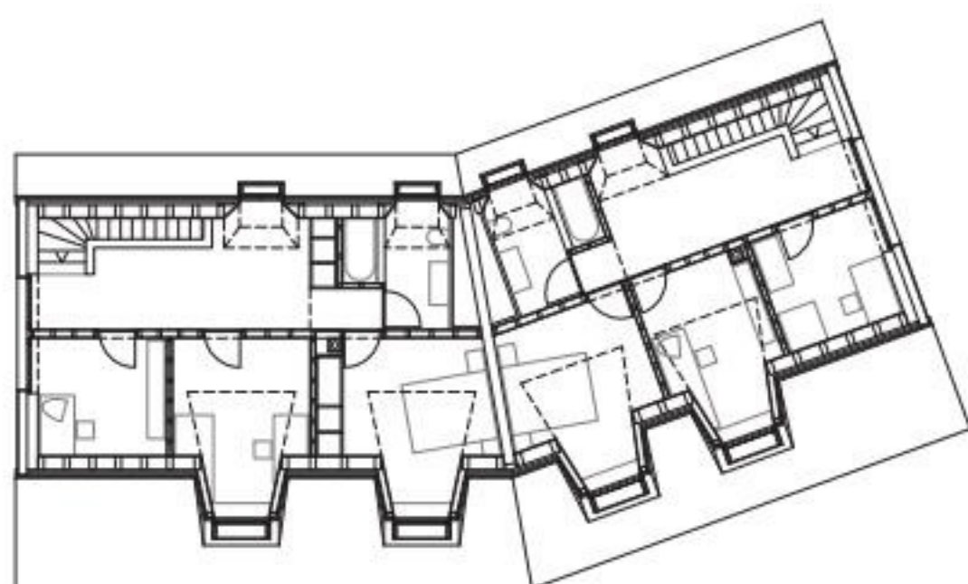
Niveau +1
